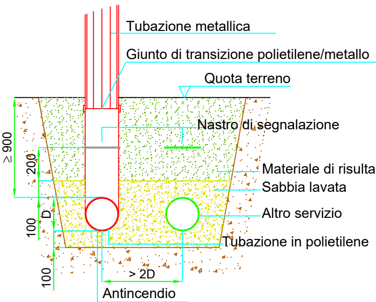
PARTICOLARE TUBAZIONE INTERRATA
