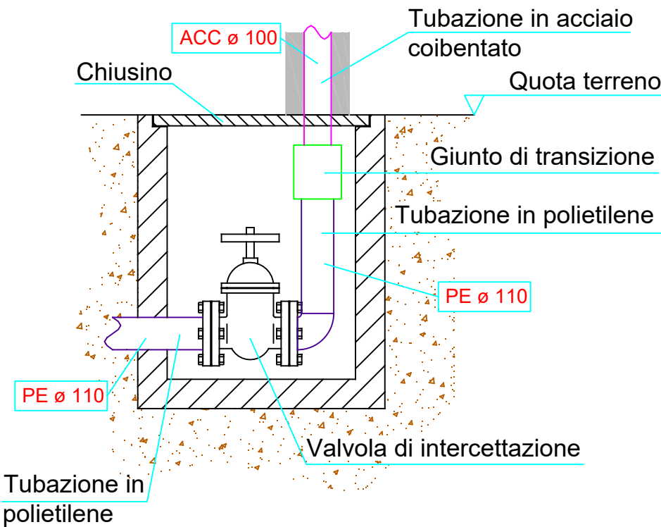
PARTICOLARI SCAVI
