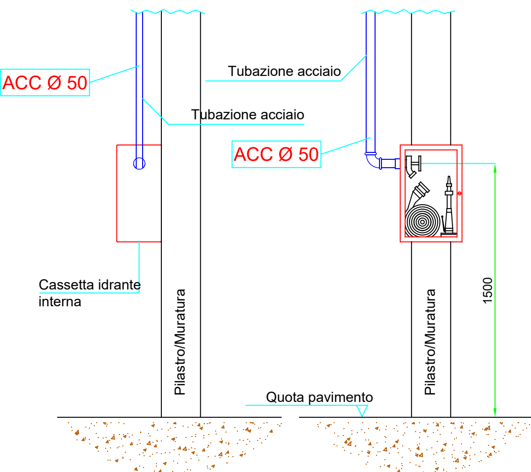
PARTICOLARE B ALLACCIO SU PILASTRO/MURATURA IDRANTE UNI 45 ALIMENTAZIONE DA RETE AEREA
