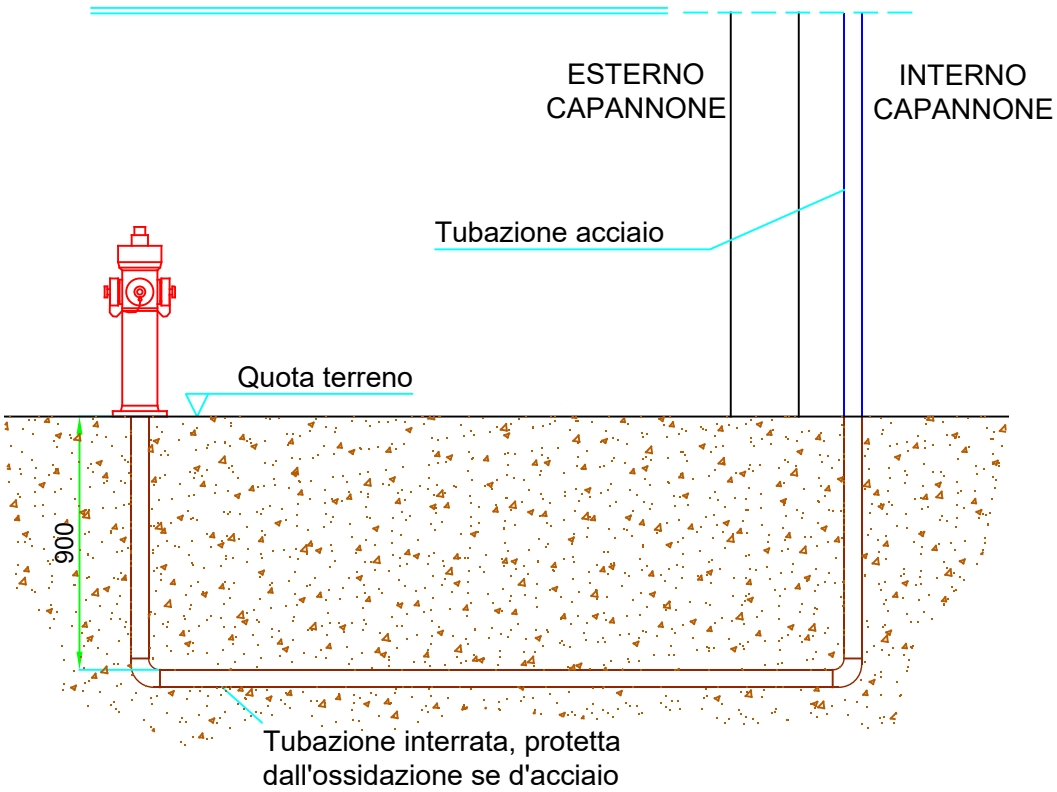
PARTICOLARE IDRANTE A COLONNA SOPRASUOLO UNI 70 ALIMENTATO DA LINEA AEREA COLLEGAMENTO SOTTERRANEO
