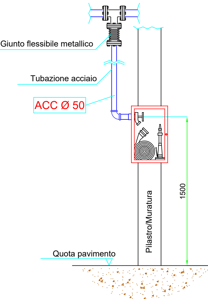
PARTICOLARE A ALLACCIO SU PILASTRO/MURATURA IDRANTE UNI 45 ALIMENTAZIONE DA RETE AEREA
