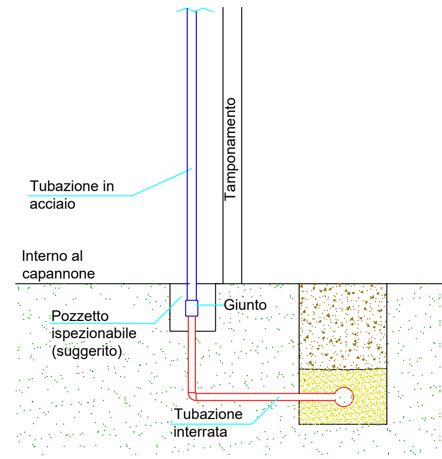
PARTICOLARE COLONNA MONTANTE INTERNA ALIMENTAZIONE DA RETE INTERRATA
