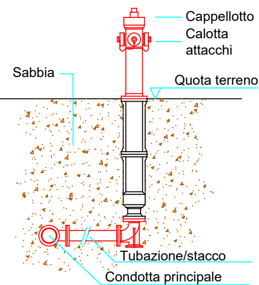
PARTICOLARE IDRANTE A COLONNA SOPRASUOLO UNI 70 ALIMENTATO DA LINEA INTERRATA
